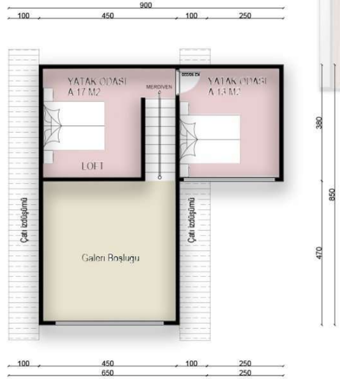
Loft Kat Planı
